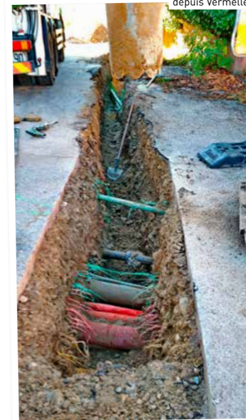
Réalimentation chateau d'eau depuis Vermelle - CAPI
